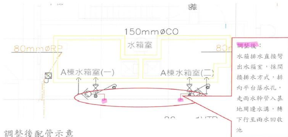
屋頂水箱排水建議調整前後對照示意圖
