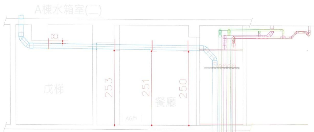
各棟屋頂水箱溢流排水管剖面示意圖
